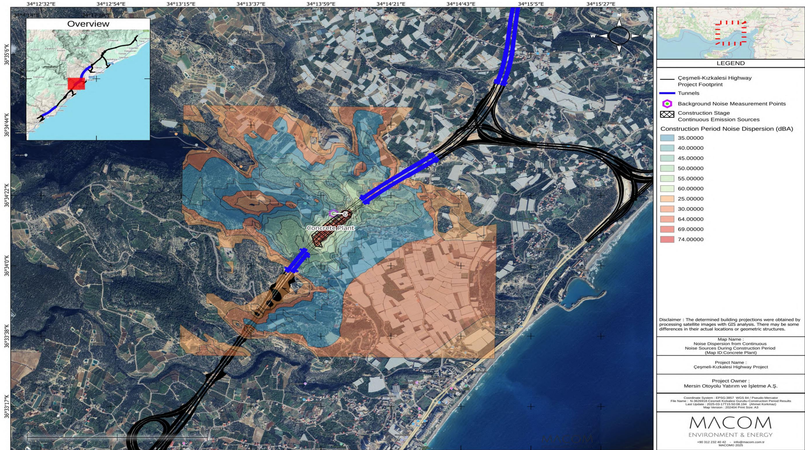
Şekil 7-5 Arazi Hazırlık ve İnşaat Döneminde Proje Güzergahı Boyunca Beton Santrali Konumu için Gürültü Dağılım Haritası
