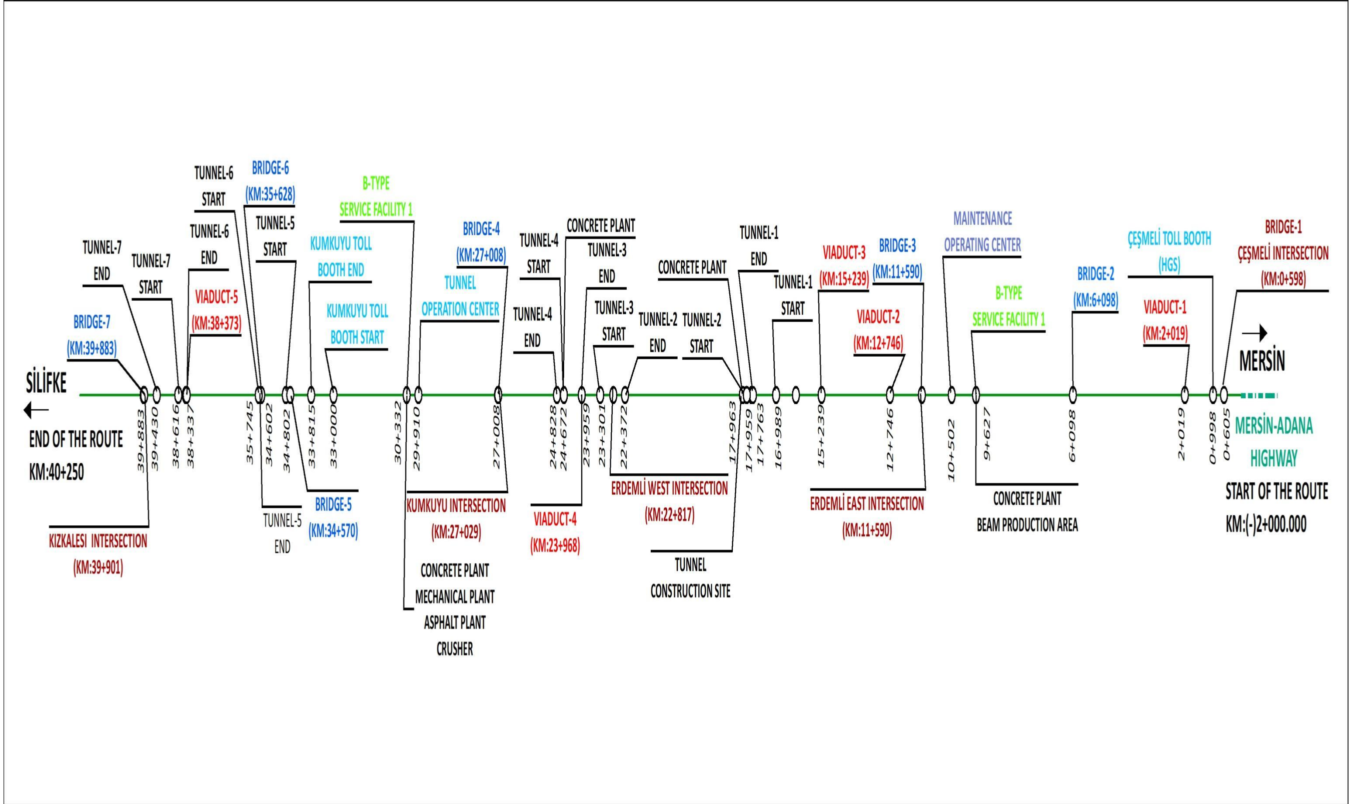
Şekil 3-2 Proje Güzergahı
