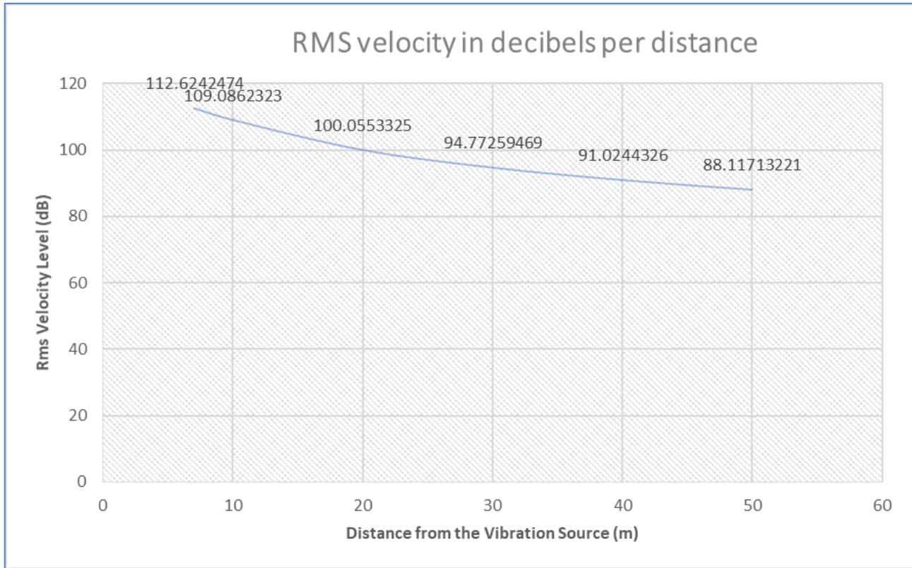
Şekil 7-9 Tüm inşaat ekipmanlarının titreşim seviyeleri
