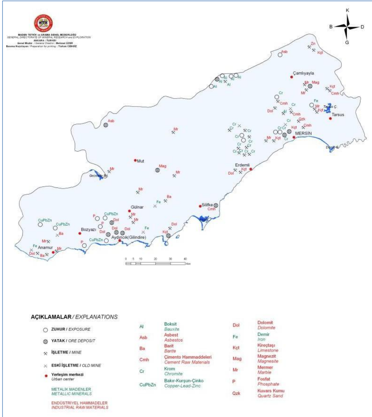
Şekil 10-1 Mersin İli Maden Haritası [32]
