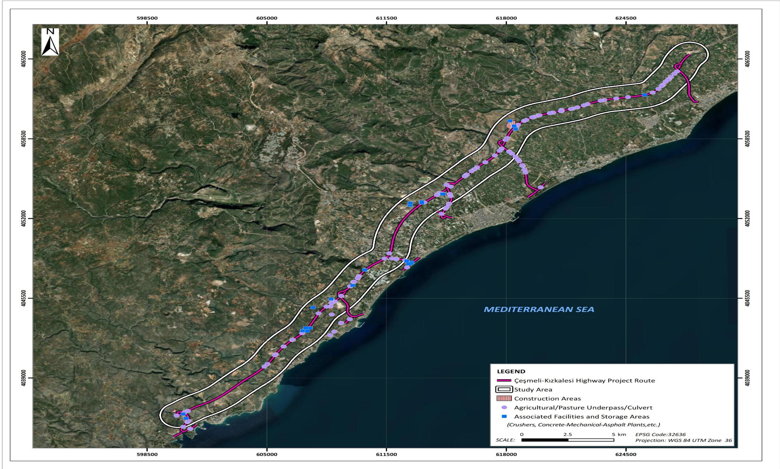
Şekil 6-11 Tarımsal Alt Geçitler ve Menfezler
