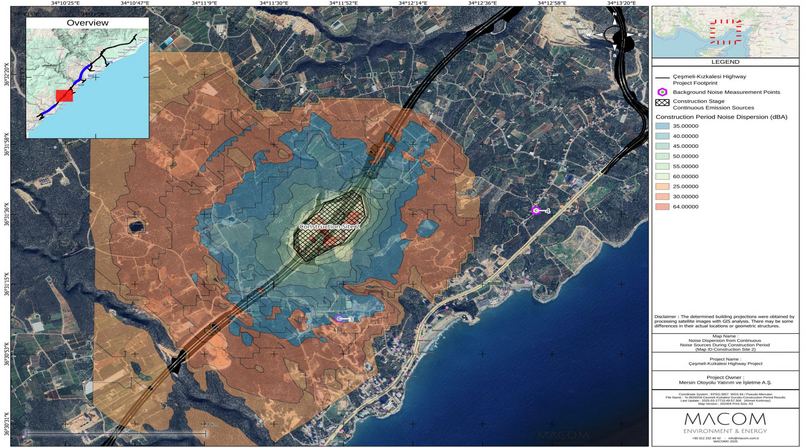
Şekil 7-4 Arazi Hazırlık ve İnşaat Döneminde İnşaat Sahası-2 için Gürültü Dağılım Haritası
