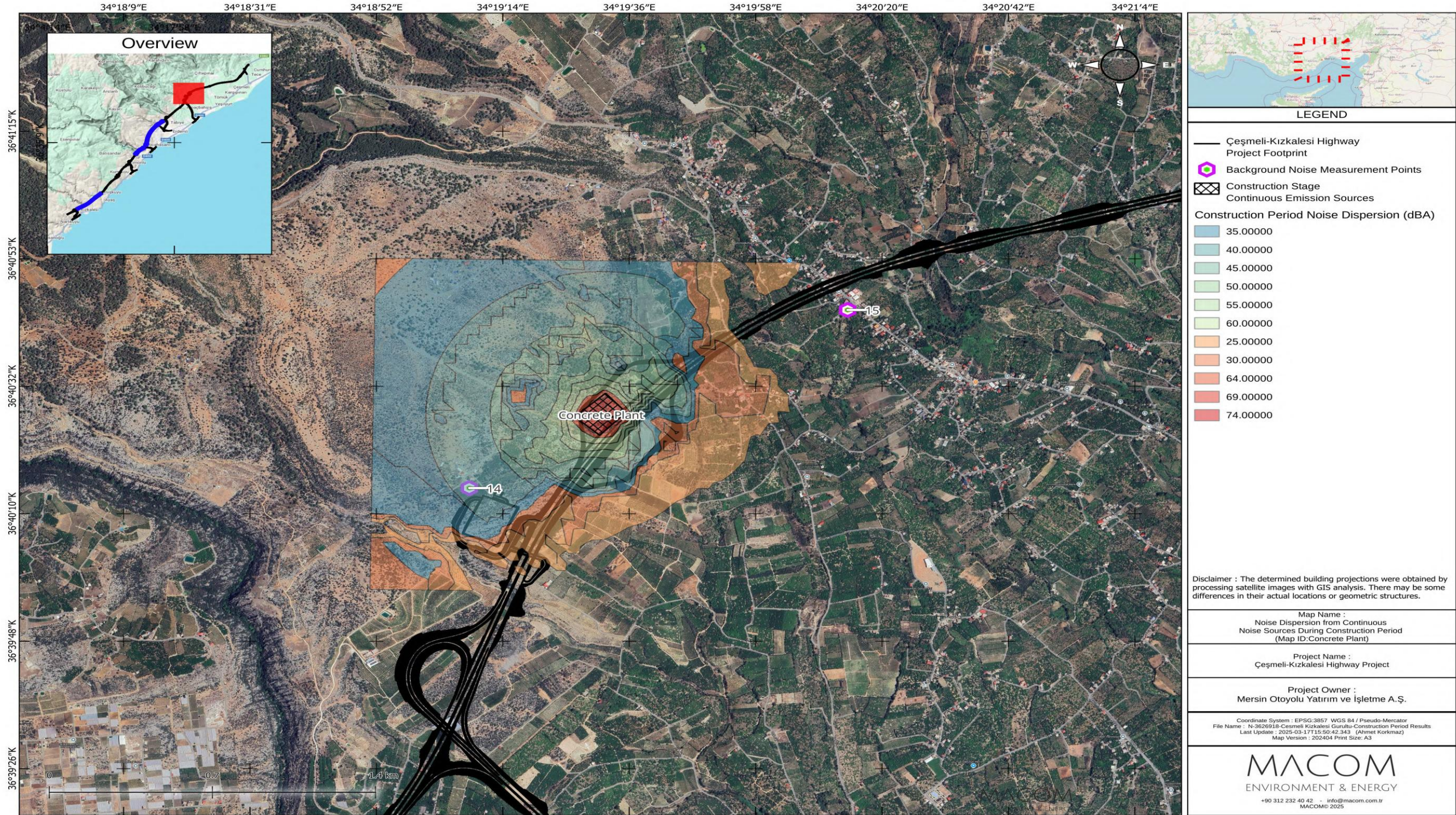
Şekil 7-8 Arazi Hazırlık ve İnşaat Döneminde İnşaat Sahası-3 için Gürültü Dağılım Haritası
