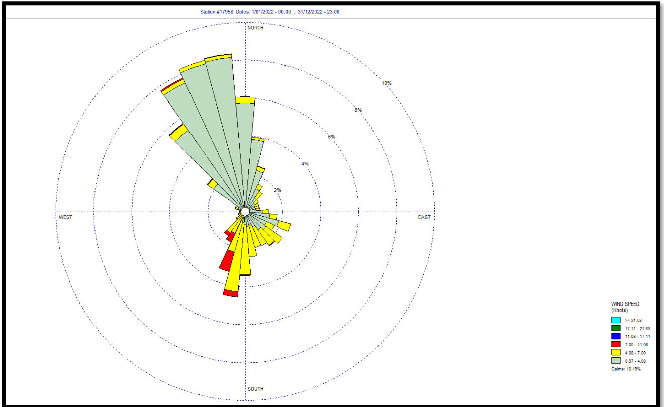
Şekil 8-4 Rüzgar Hızına Göre Esme Yönünde Rüzgar Gülü
