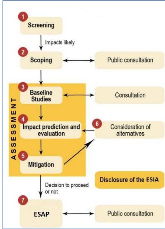
Şekil 5-1 ÇSED Süreci
