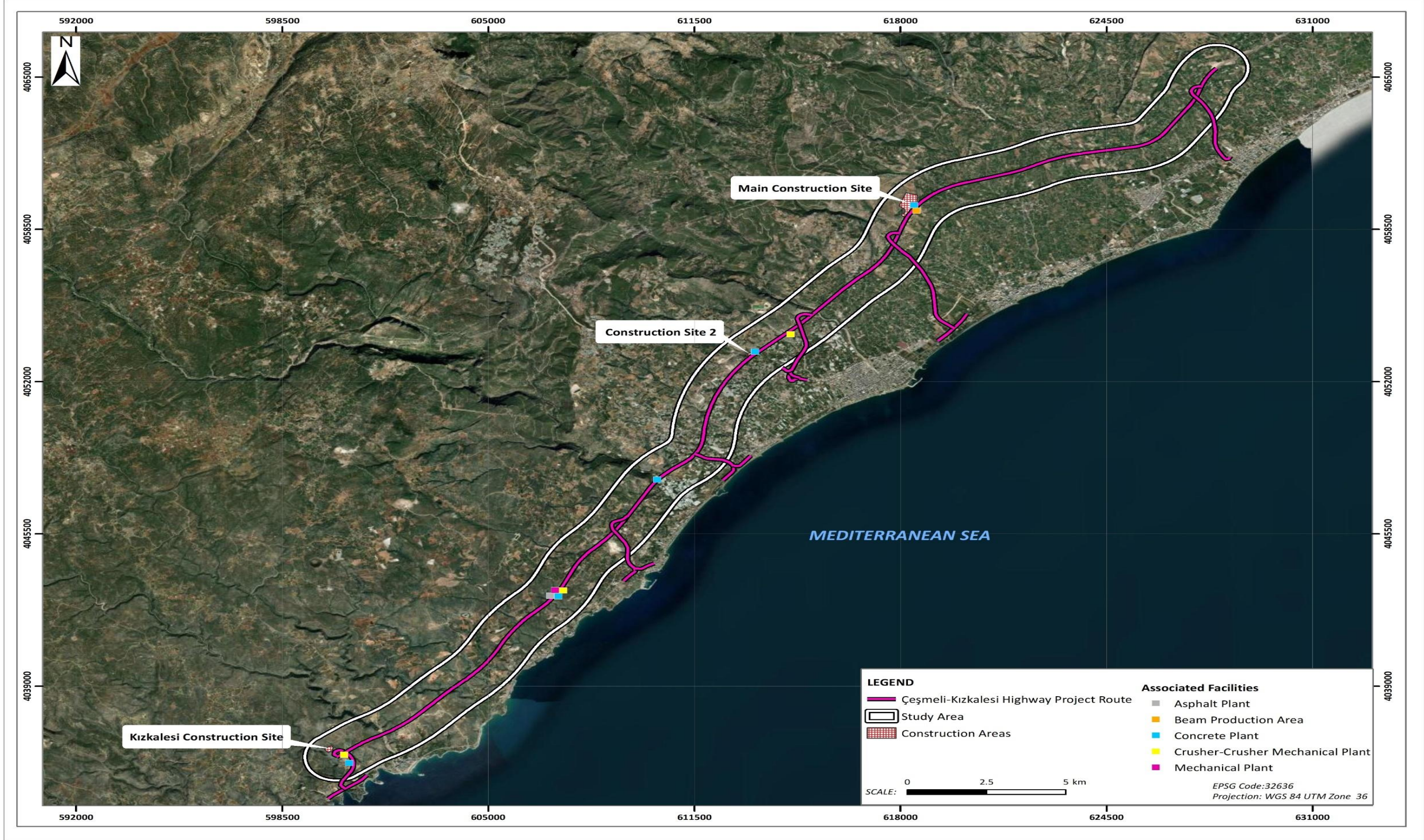
Şekil 6-13 Proje Güzergahı Üzerindeki Geçici Tesislerin ve Şantiyelerin Konumları
