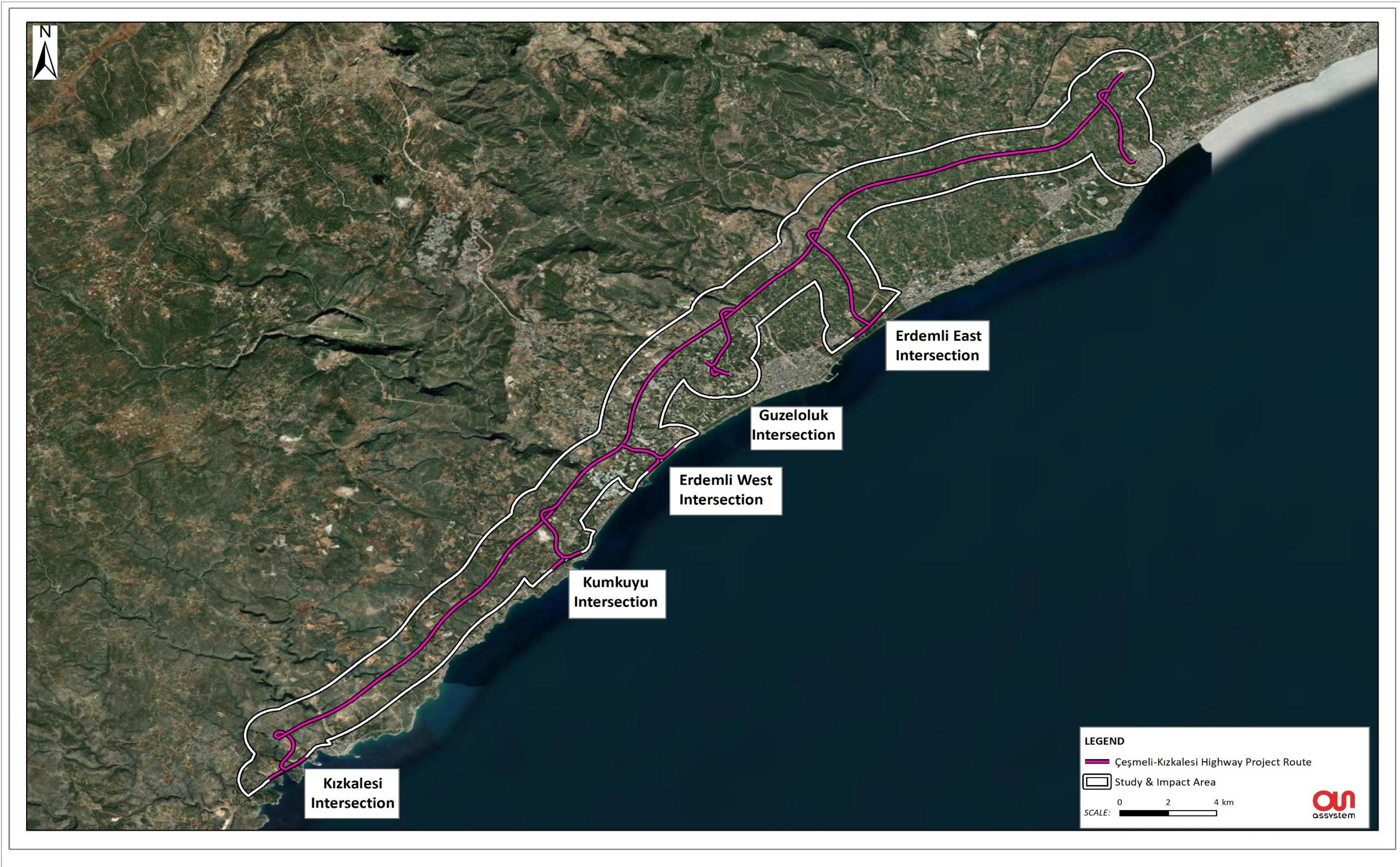
Şekil 3-1 Ana yol ve bağlantı hatları (Kaynak: Proje ÇSED, 2024)
